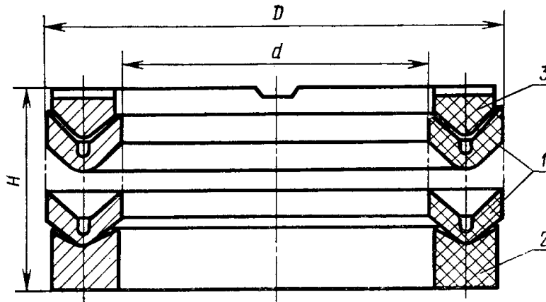
1—шеvronная манжета; 2—нажимное кольцо; 3—опорное кольцо
